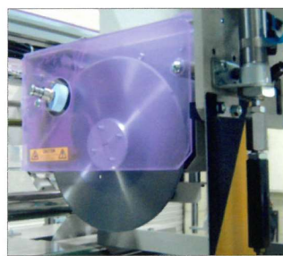
上下分離カッター
