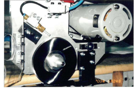
高速回転式カッター
