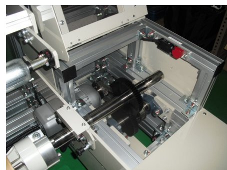
直駆動巻取機構
