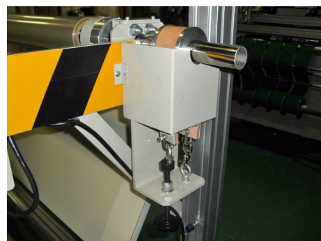
原反ブレーキ(調整式)
