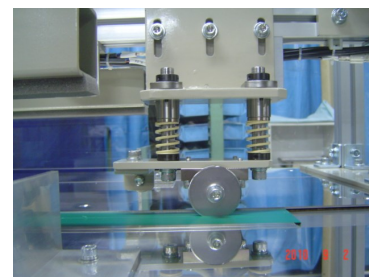
カッターユニット
