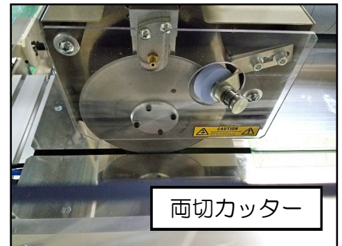
裁断装置本体 (吐出テーブル側)
